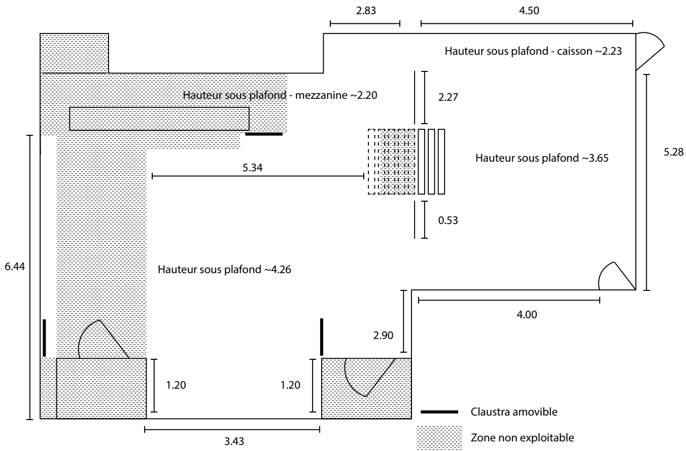
Plan schématique Hall et salle d'exposition A.B.C.
